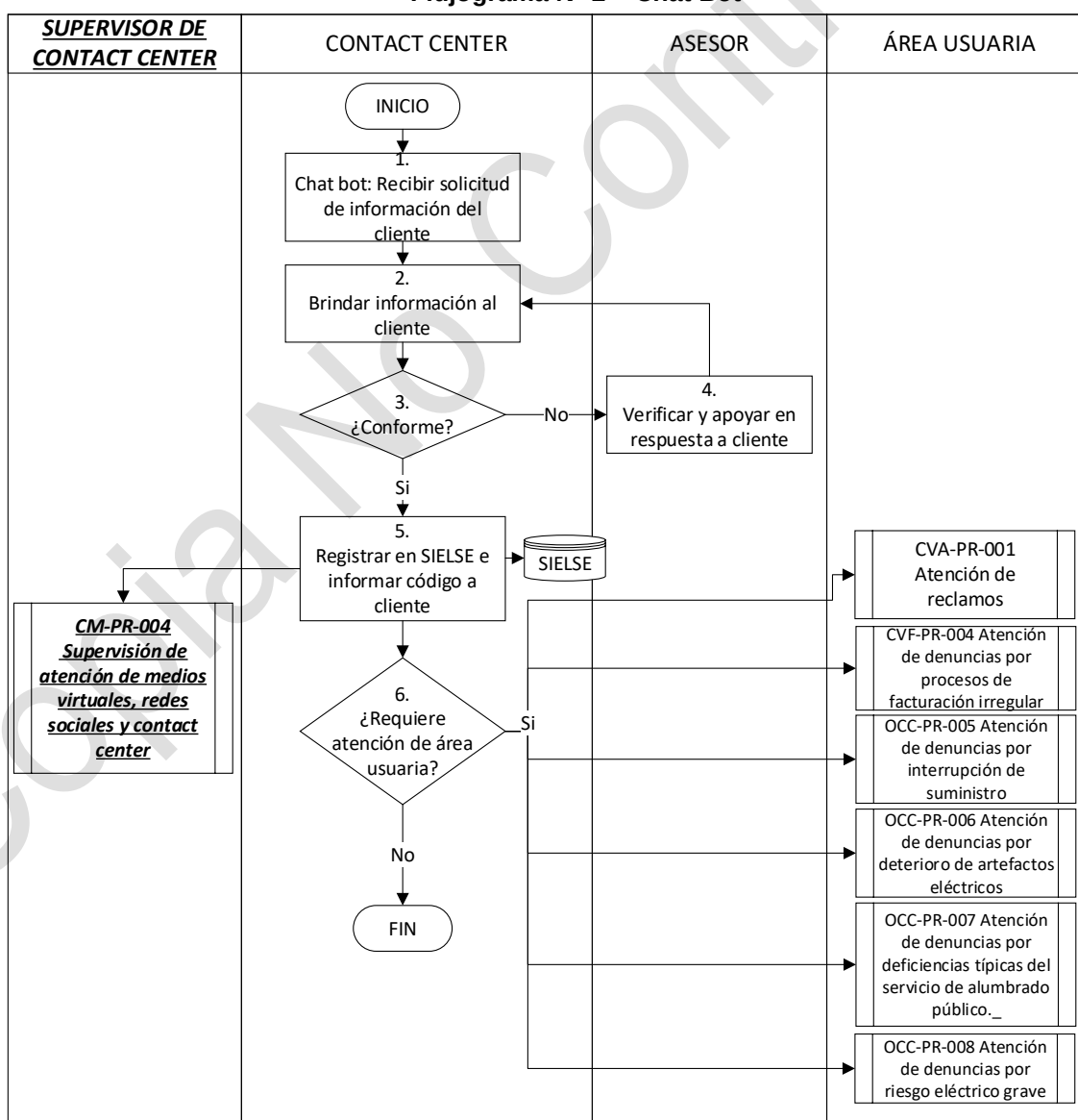
Flujograma N° 2 – Chat Bot
