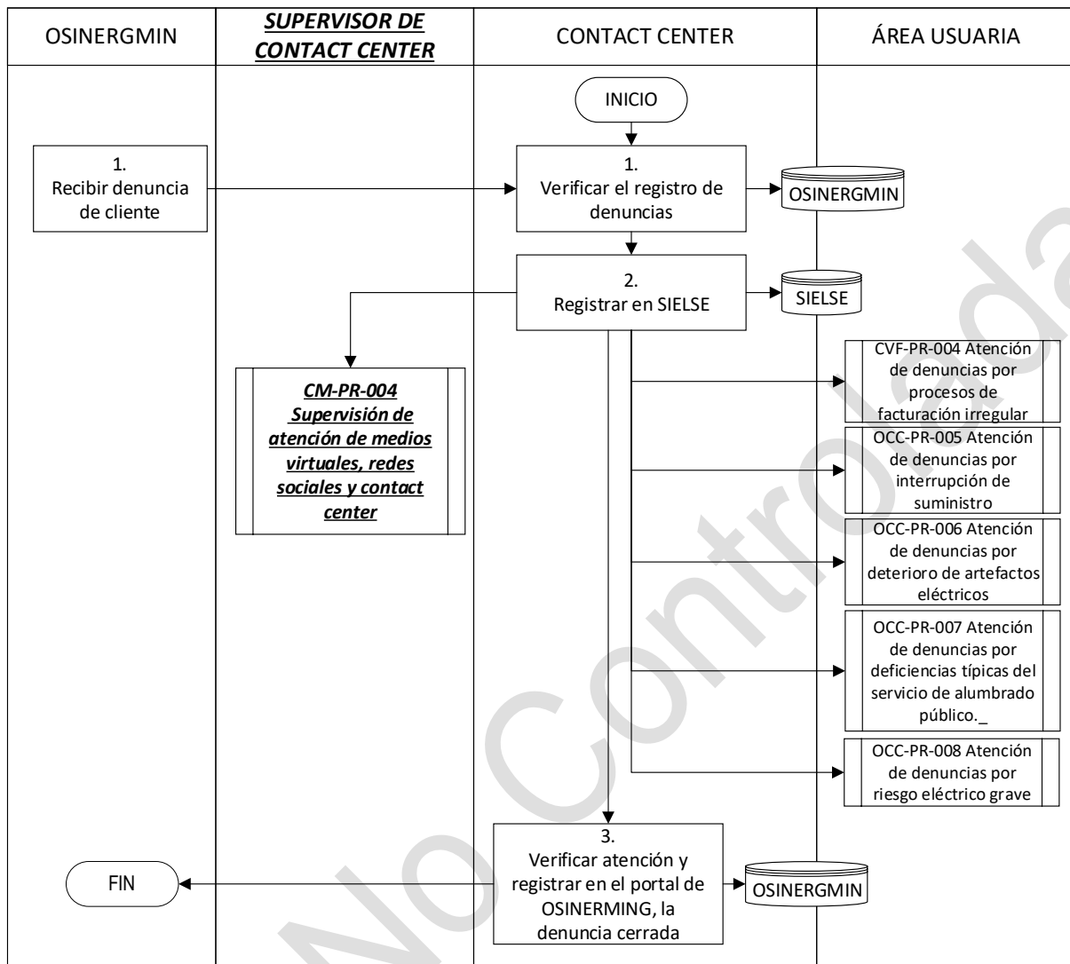
Flujograma N° 3 - Tukuy Ricuy
